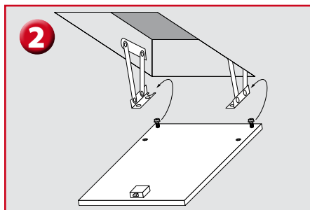
Montage Luke mit Einhanghilfe
