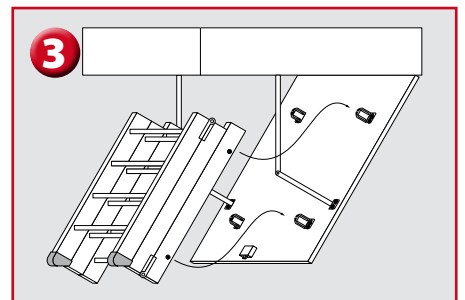
Montage Treppenteil
